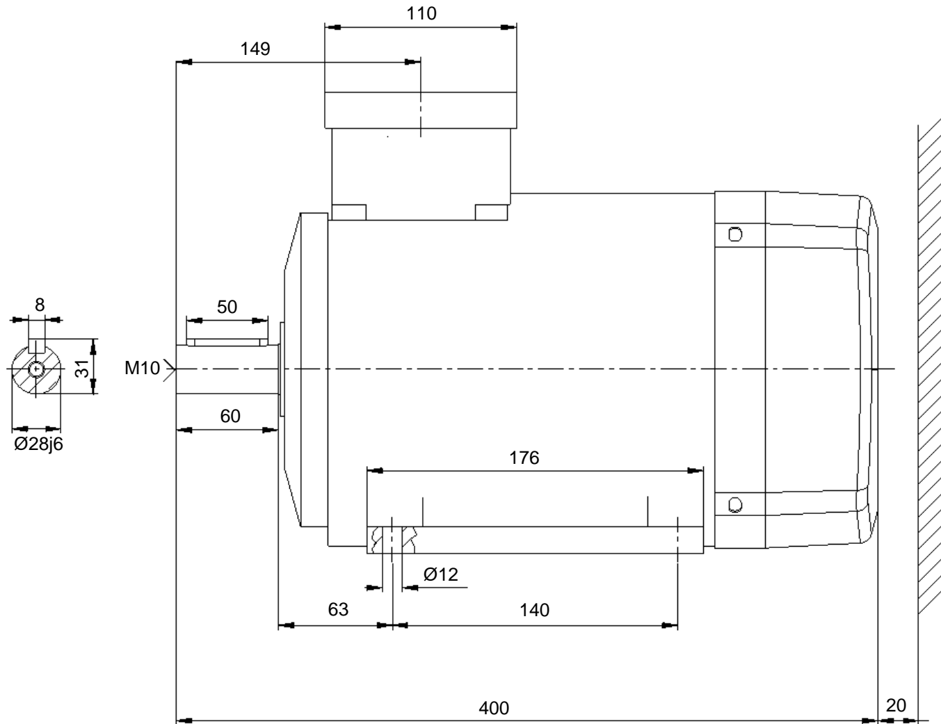
Maßblatt - #303422 - KTE3 100 L 4 KT FL IE3 in Angebot An162997 Position 1 Kabelverschraubung: 2x M25x1,5
